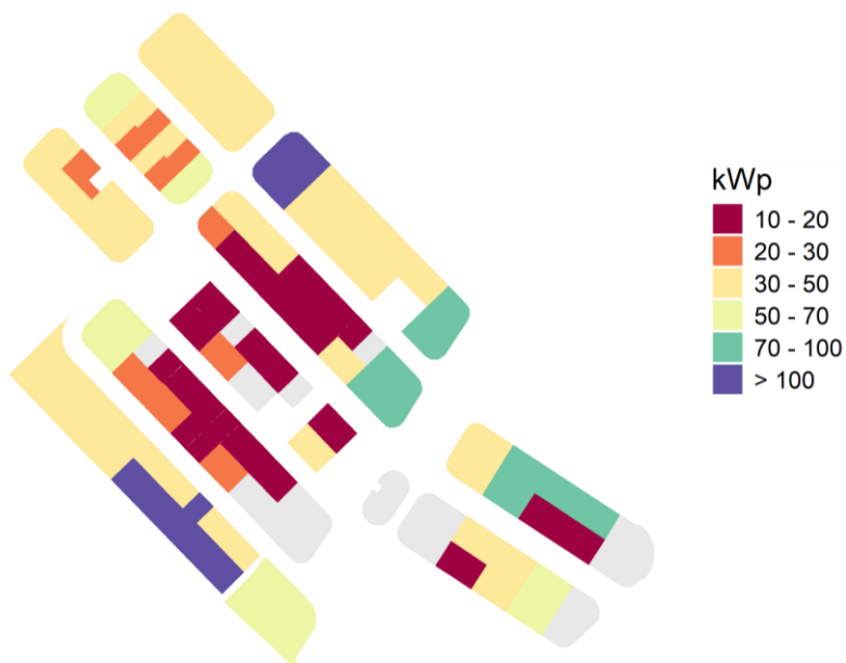
Figura 8. Potencia instalable óptima asignada a los edificios con usos de tipo industrial.
