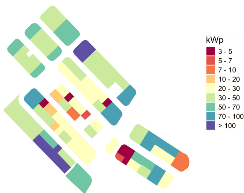
Figura 4. Potencia instalable óptima para todos los edificios del polígono.
